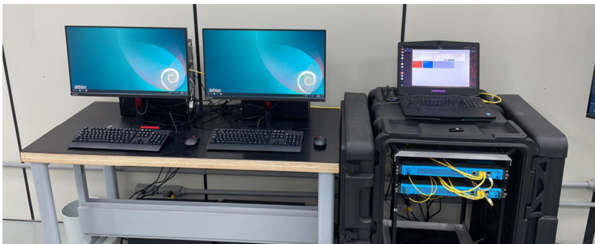
Sistema Cerberis (ID Quantique) de troca de chaves quânticas, entrando em operação
