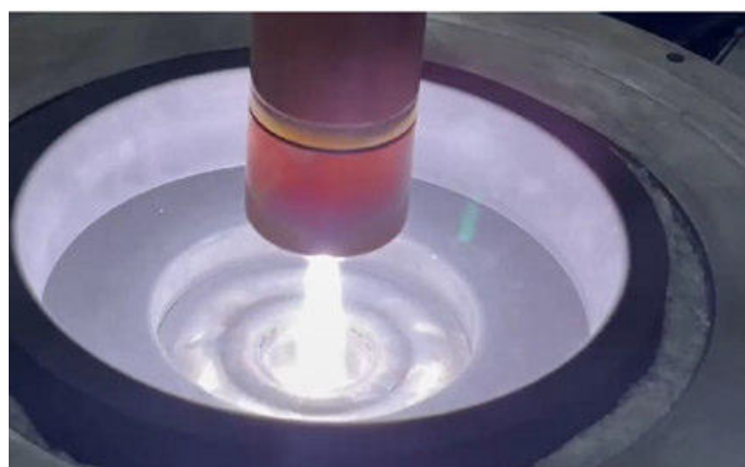
Imagens da Região de Formação do Arco Transferido da Tocha de Plasma (Catodo) para o Anodo
