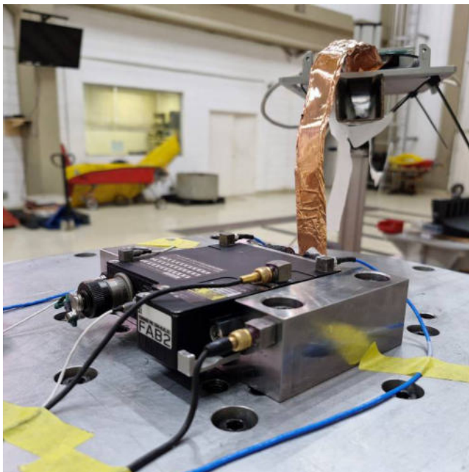
Ensaio Ambientais do Criptocomputador Nacional CM4-B. Ensaio de vibração
