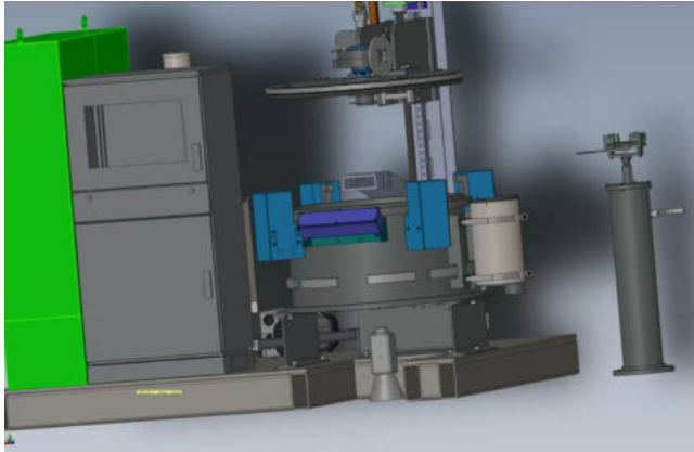
Equipamento Spin Pit para ensaios de sobrevelocidade, fadiga ("LCF") e implosão intencional ("burst") de rotores
