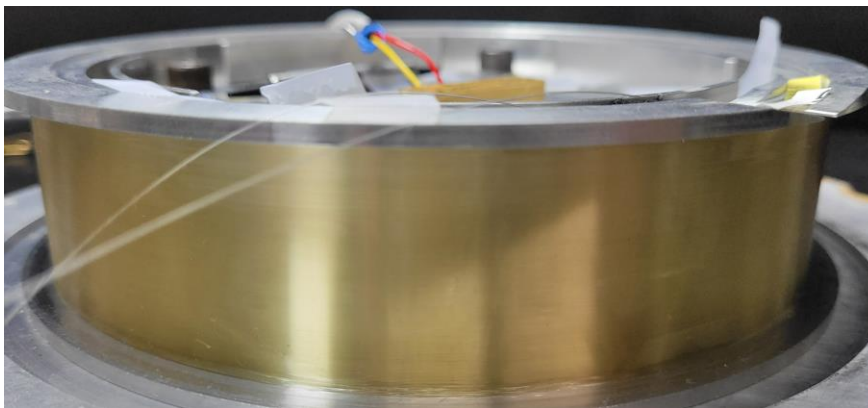
Giroscópio a Fibra Óptica construído no Projeto IFO
